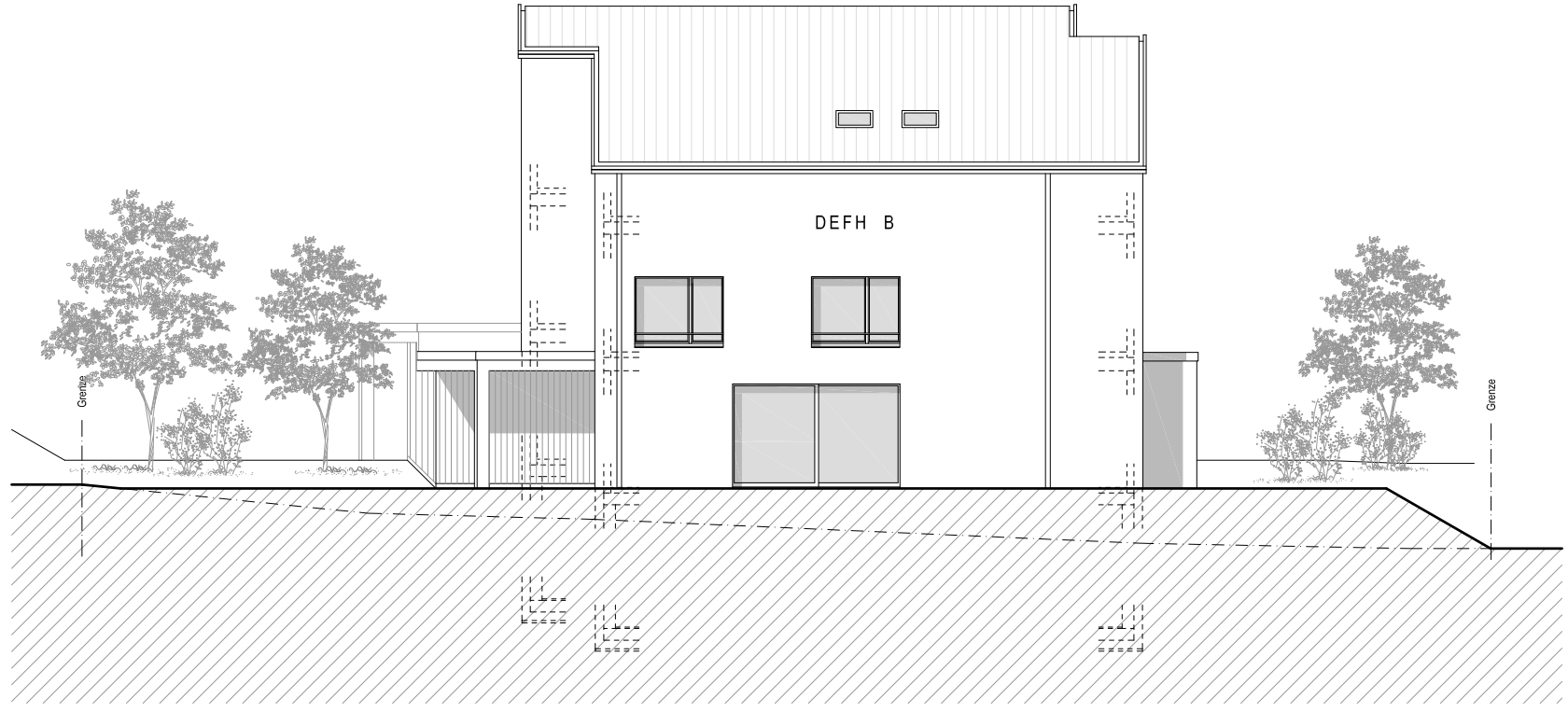
Ostfassade
