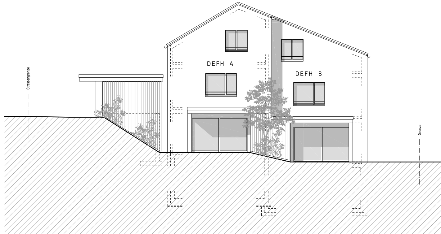
Südfassade
