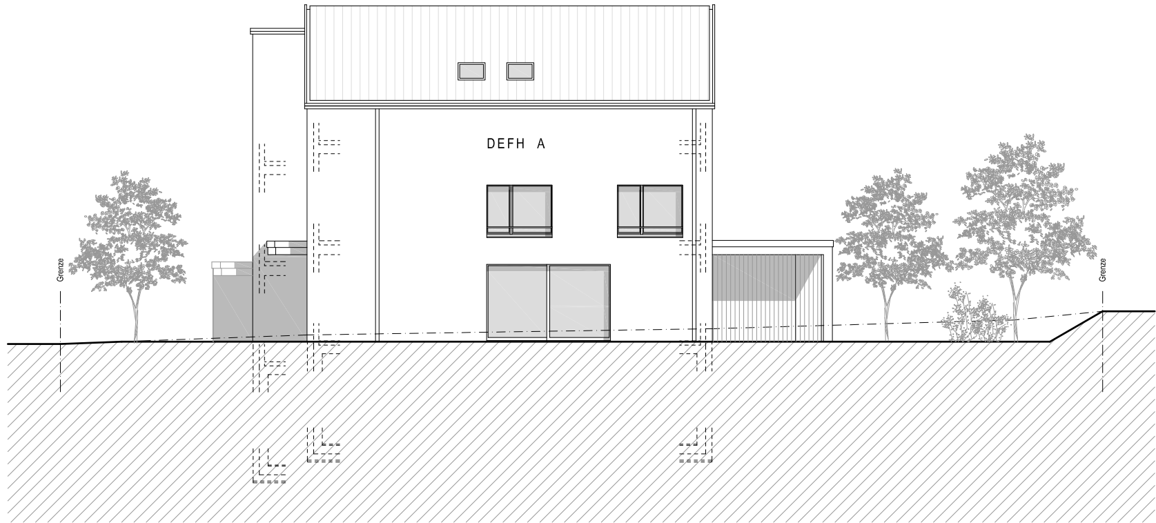
Westfassade
