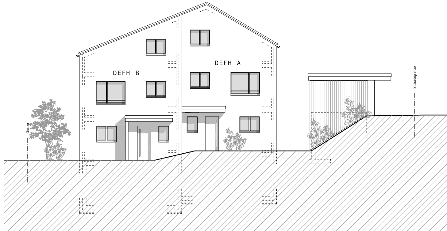
Nordfassade
