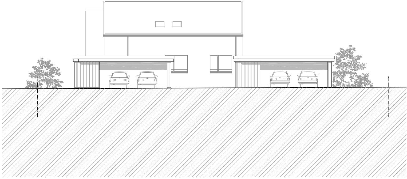
Westfassade
